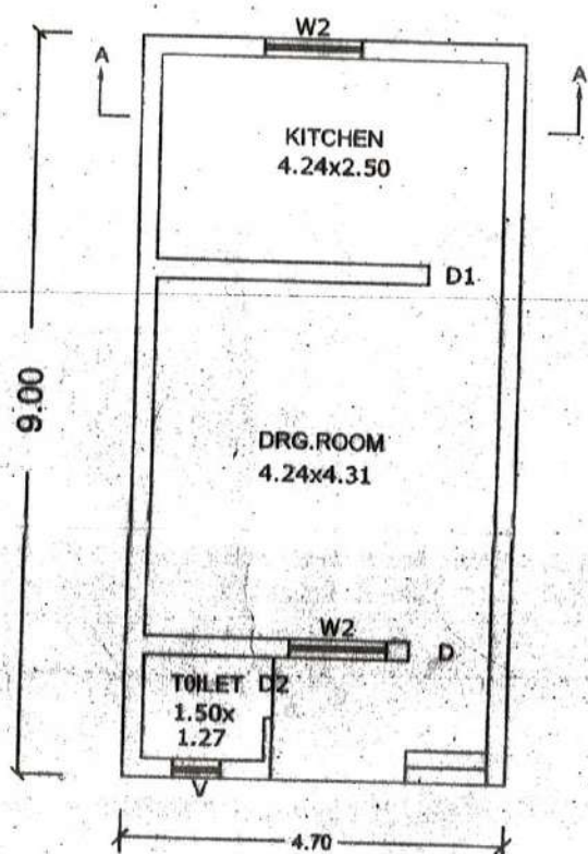
G.F. & F.F. PLAN
