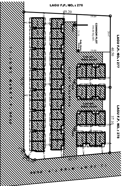
LAY OUT PLAN SCALE: 1 CM = 3.00 MT
