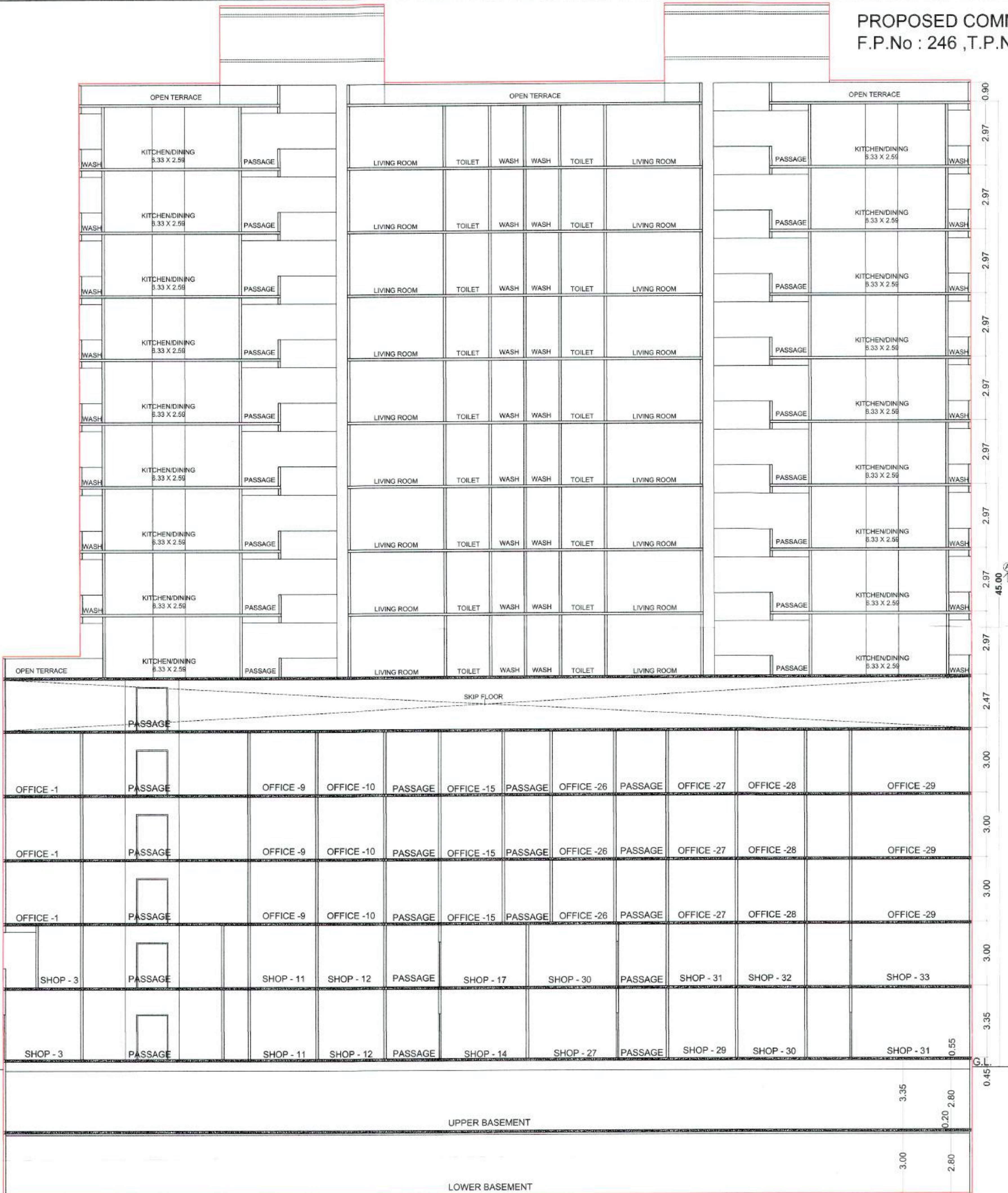
SECTION : A - A
