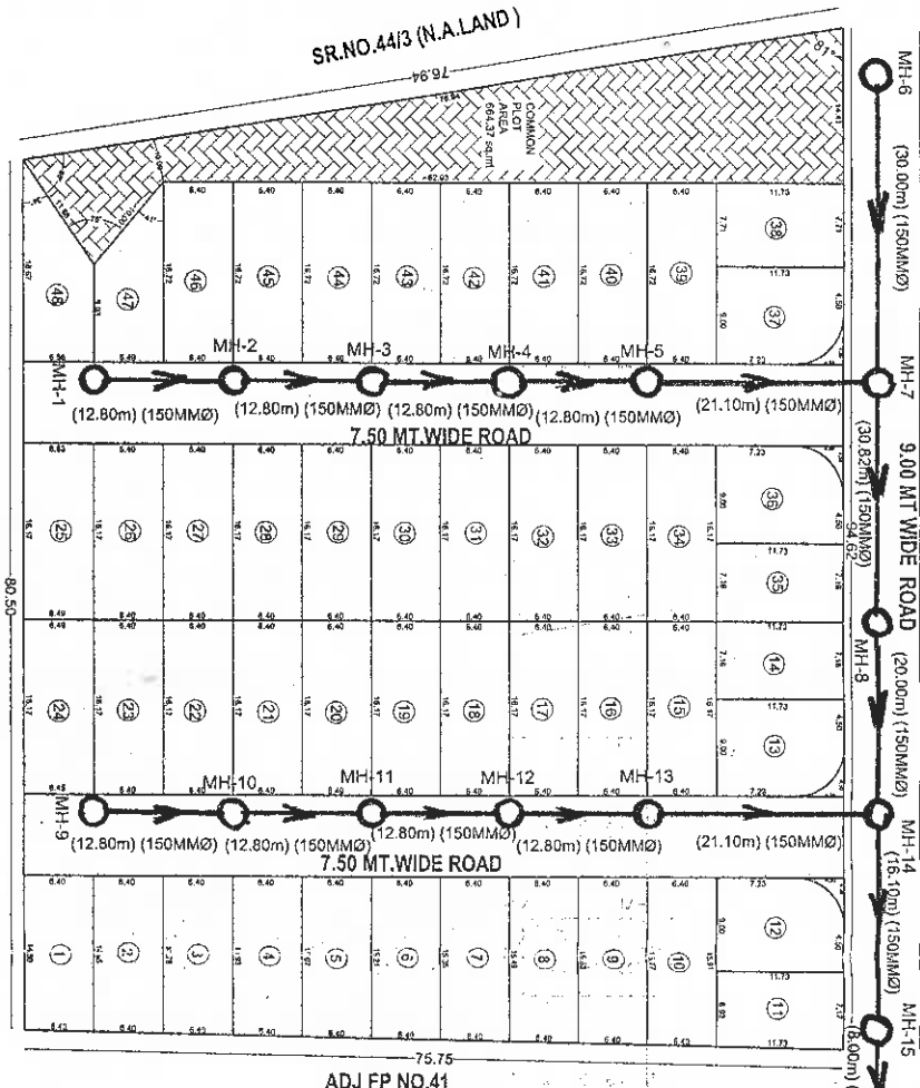
LAY OUT PLAN (SCALE: SR.NO.45/2 D (N.A.LAND))
