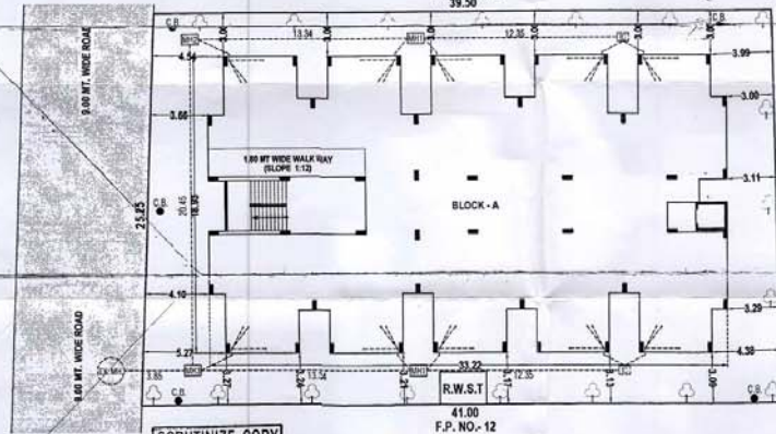
LAYOUT PLAN SCALE: 1 CM = 2.00 MT
