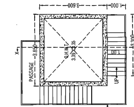
CHWT PLAN
