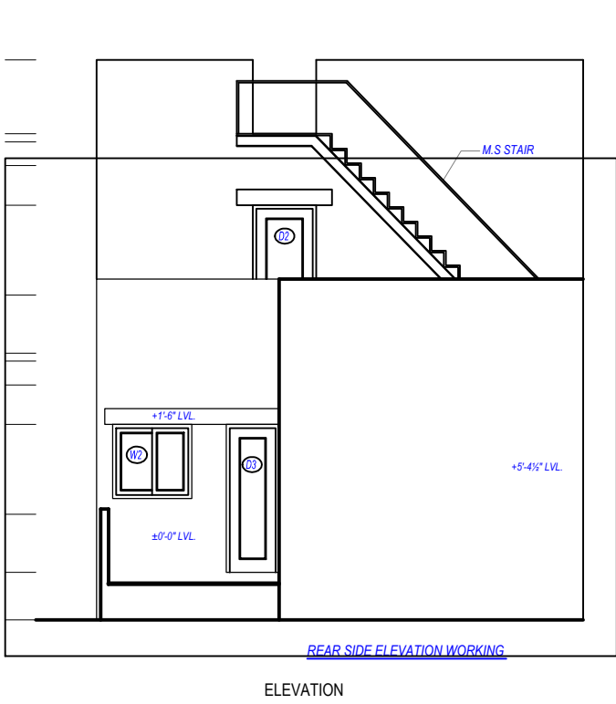
ELEVATION
