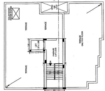
TERRACE PLAN SCALE: 1/8" = 1'-0"
