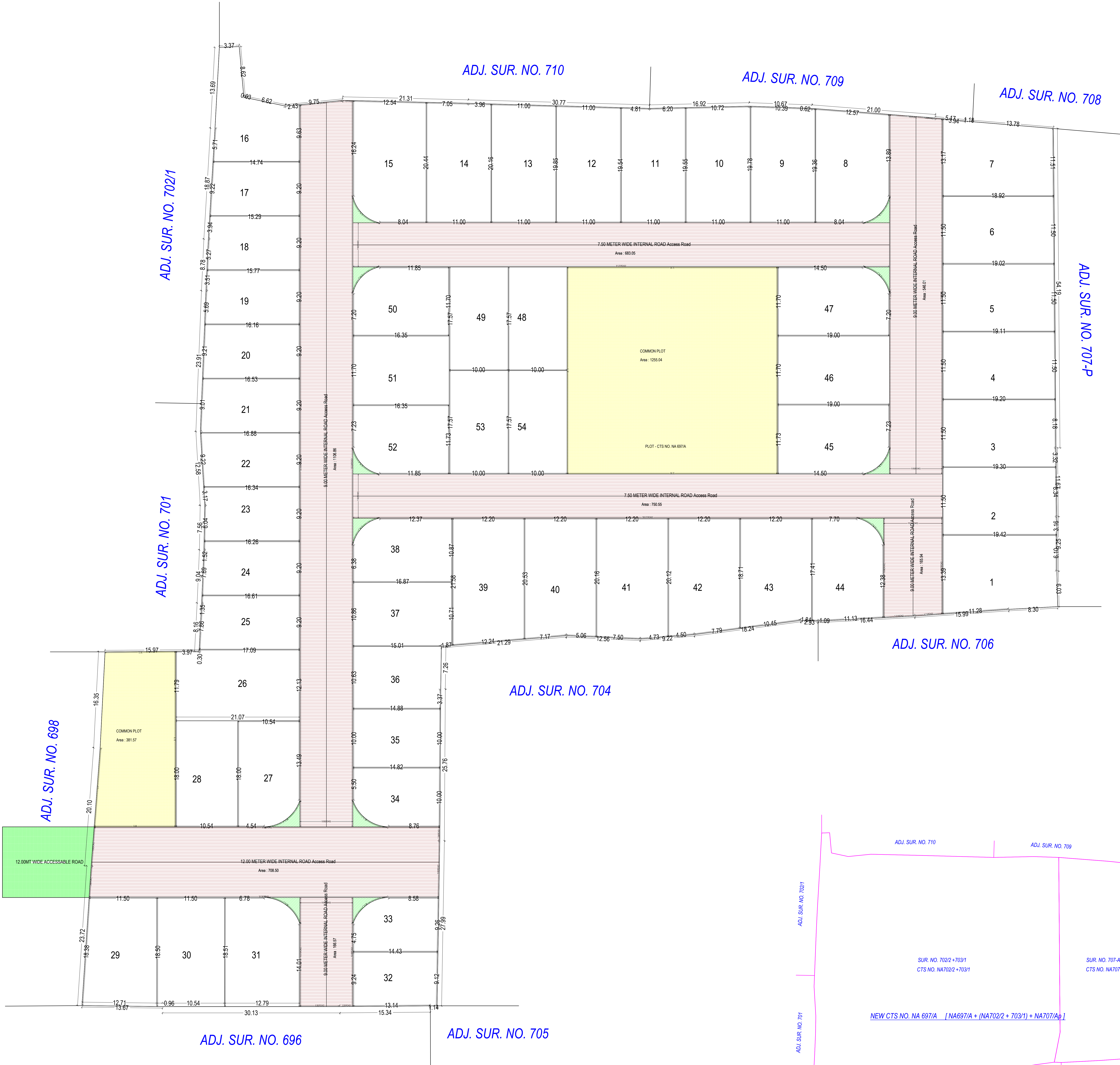
SITE PLAN (Scale - 1:200)
