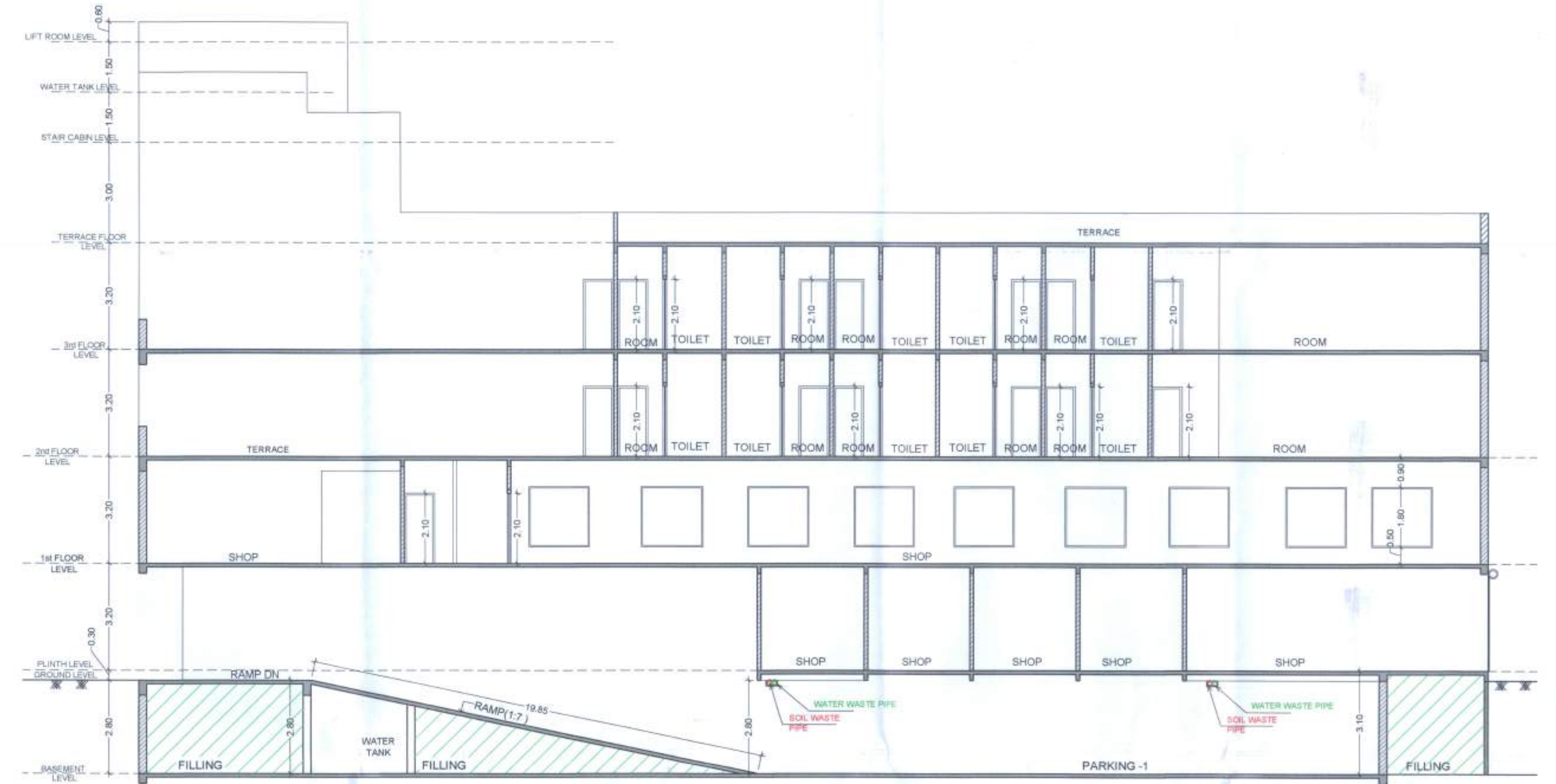
SECTION B-B SCALE: 1/10M = 1.0 MT.
